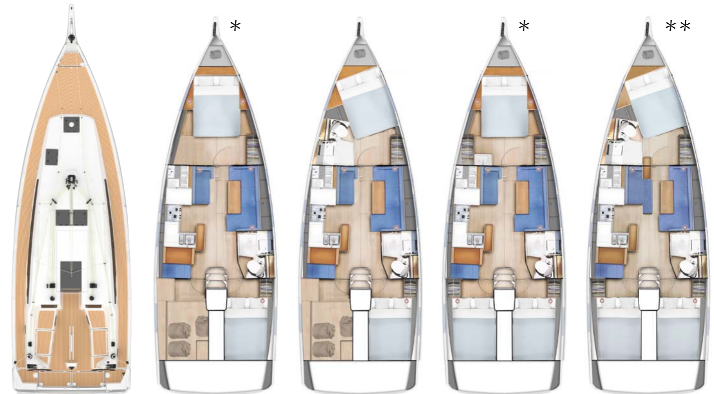
*Optional dressing and furniture with private sink to portside (in forward cabin) / Dressing et meuble avec lavabo privatif à bâbord (dans la cabine avant) en option. **Lifting keel version / Version quille relevable.
